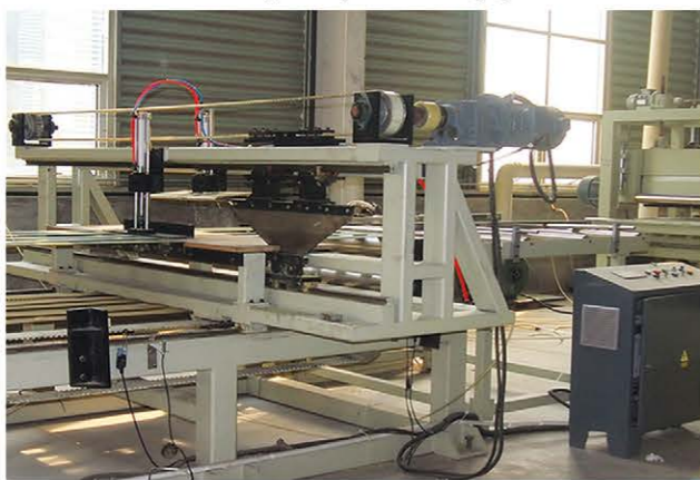
XPS-CO2 extrusion line
