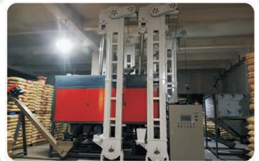
← 硅胶橡胶分离机 RUBBER SEPARATOR
